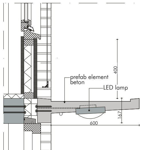
Verticaal detail nieuwe luifel. Tekeningen: Vanschagen Architecten.
