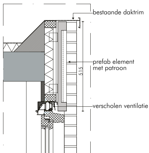
Verticale doorsnede bij dakrand.
